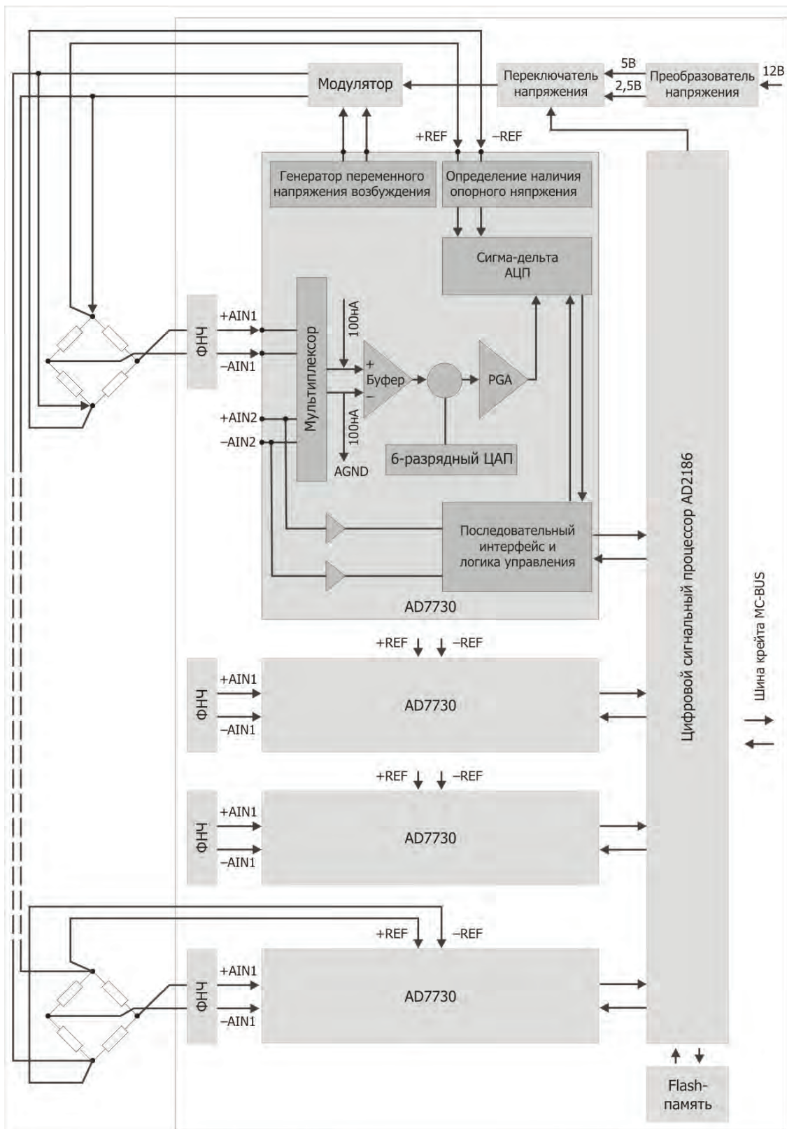
Рисунок 1.22 — Функциональная схема модуля MC-212
