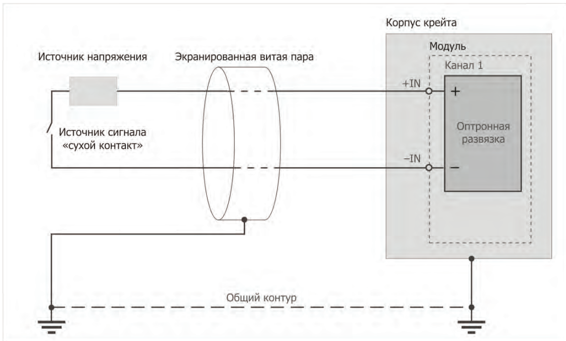
Рисунок 1.34 — Схема подключения источника сигнала с «сухой контакт» к модулю MC-401 (поканальная гальваническая развязка обеспечивается)
