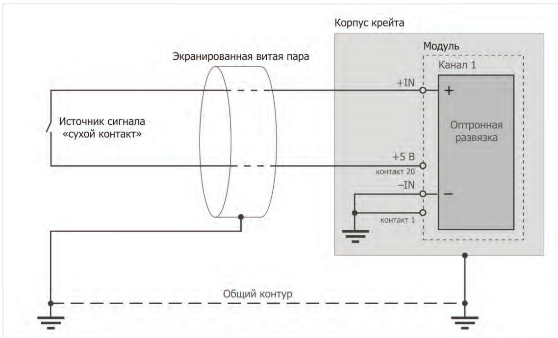
Рисунок 1.35 — Схема подключения источника сигнала с «сухой контакт» к модулю MC-401 с питанием от внутреннего источника модуля (поканальная гальваническая развязка не обеспечивается)
