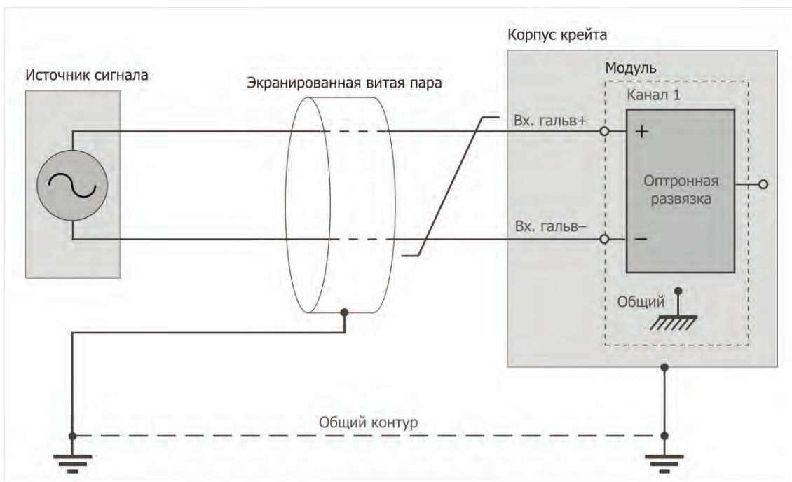
Рисунок 1.30 — Схема подключения источника сигнала к гальванически изолированным входам модуля MC-451
